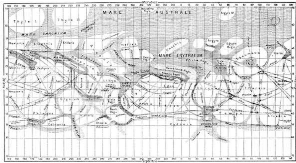
Schiaparelli Mars-térképe
