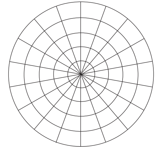
Déli jégsapka
