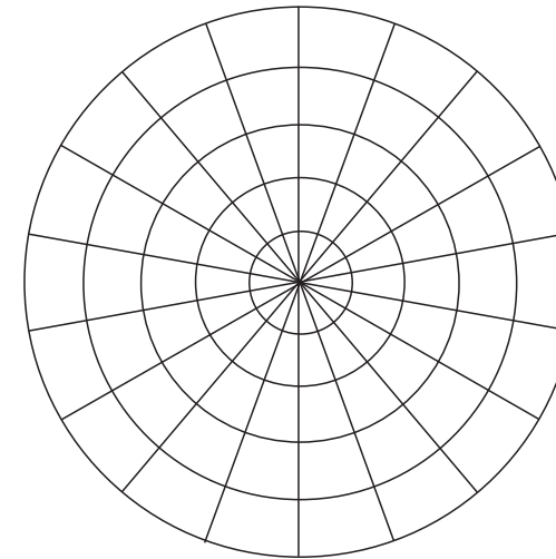
Északi jégsapka
