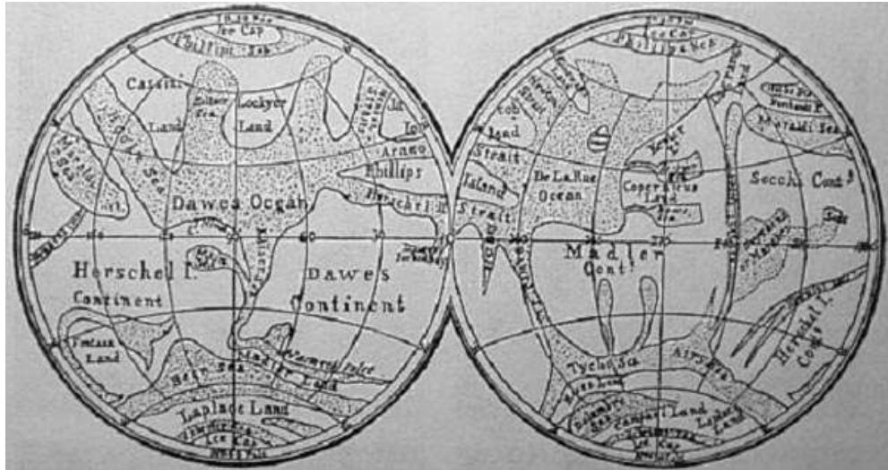
Proctor Mars-térképe
