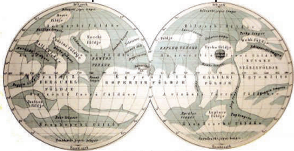
Flammarion Mars-térképe
